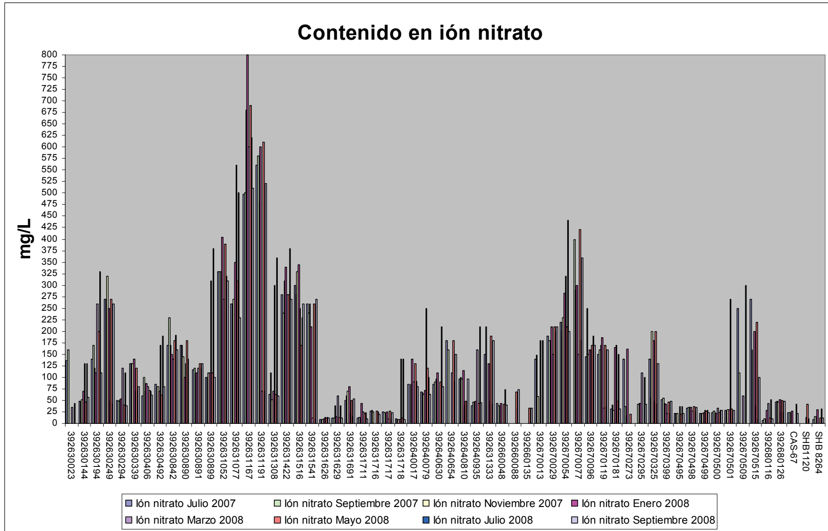
Figura 7.- Contenido en ión nitrato en los meses de Marzo, Julio, Septiembre y Noviembre de 2007 y Enero, Marzo, Mayo, Julio y septiembre de 2008.
