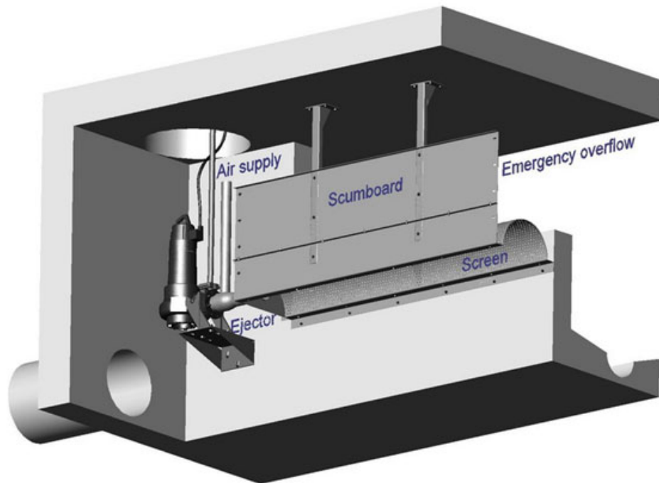
Modelo en 3-D de un tamiz de aliviadero de limpieza automática tipo PAS.
