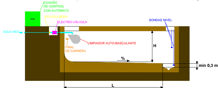
Figura 1: Circuito de llenado con agua de red.
