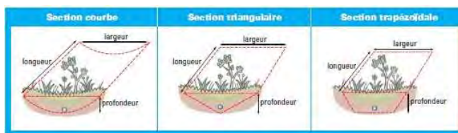
Différentes forme de noues
