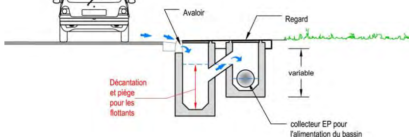
Fonctionnement d'un Regard siphonide
