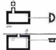
coupe longitudinale faisant apparaître l'ouverture de visite et le système de trop-plein
