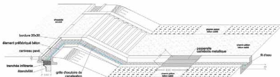
Principe de descente d'eau pluviale
