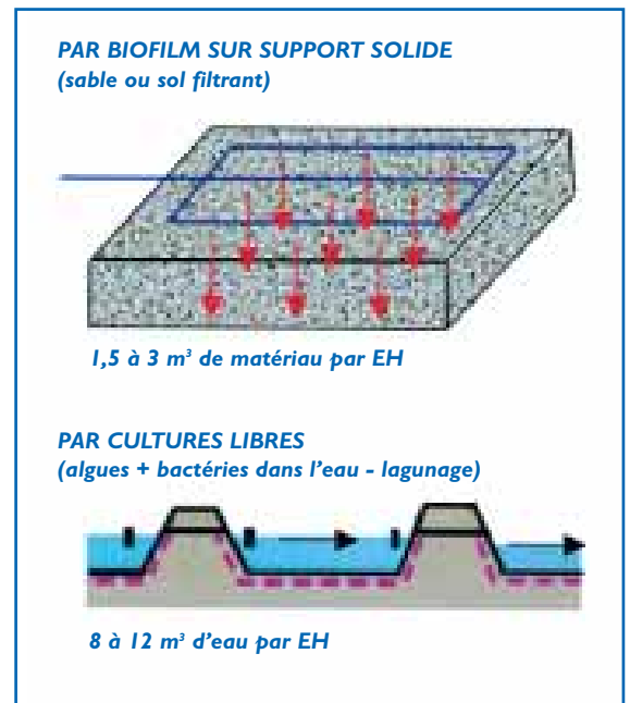
Figure n° 5 : Epuration "naturelle" extensive des eaux usées (Jean Duchemin, Commission Européenne - 2001)
