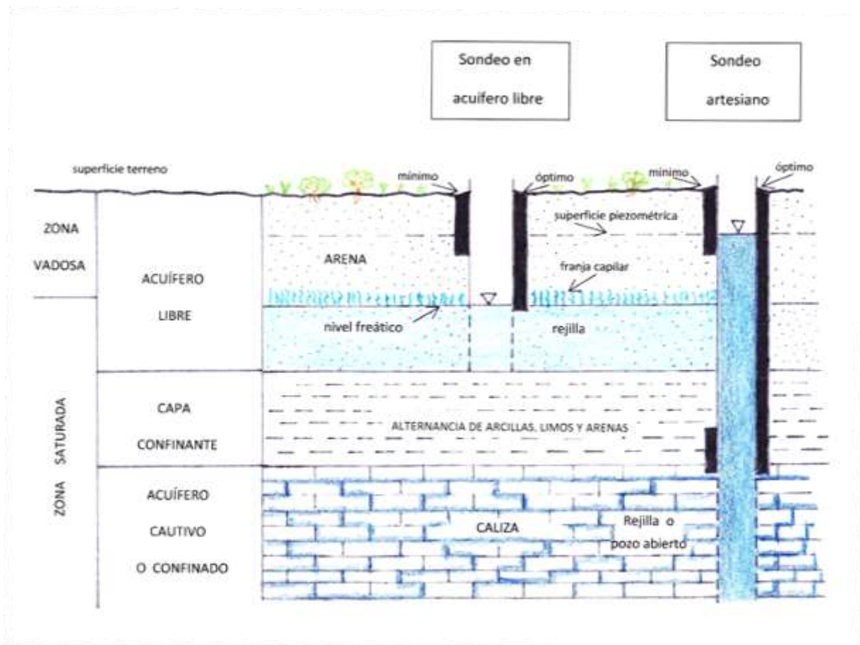
Figura 1. Esquema de cementación para acuíferos libres y confinados.
