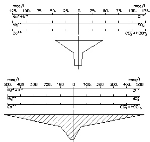
Diagrama de Stiff modificado (Rayado: cambio de escala).
